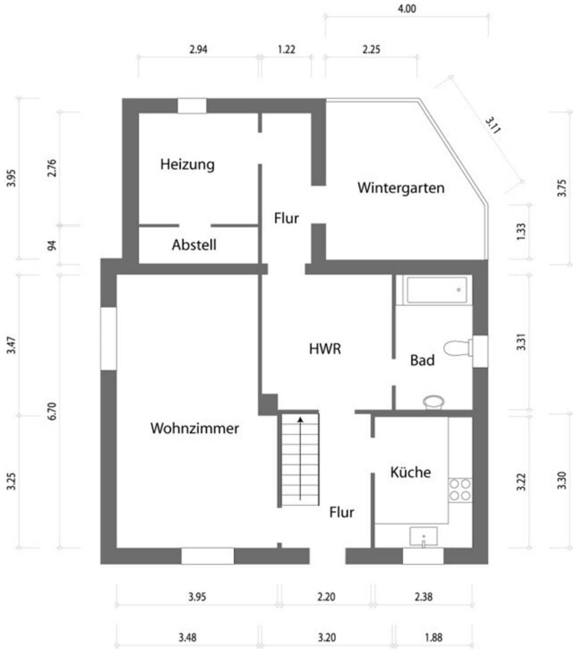
Grundriss EG
