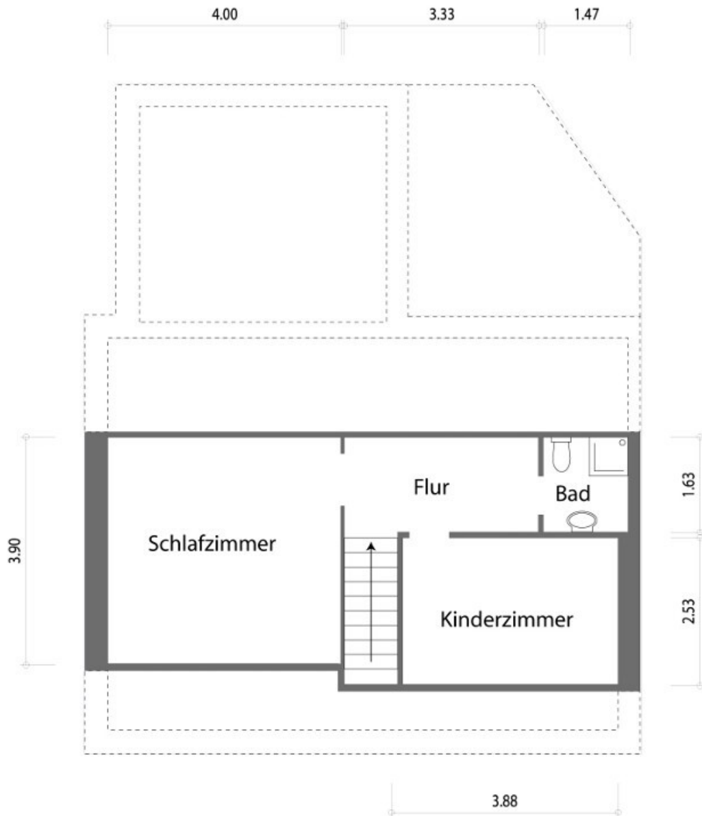
Grundriss DG
